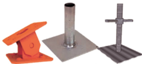
SAPATAS ARTICULÁVEIS; FIXAS OU AJUSTÁVEIS
